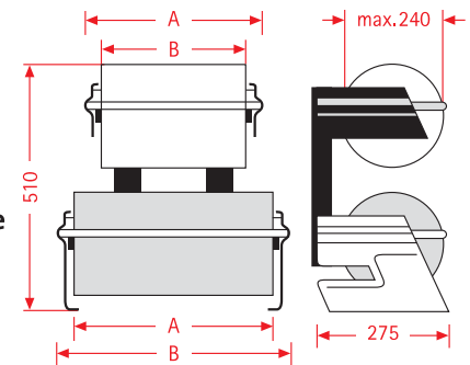
Aufsatz-Abroller dispenser attachement dérouleur superposable
