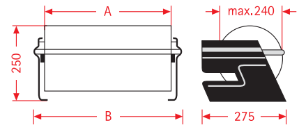
Tisch-Abroller table dispenser dérouler de table
