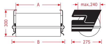
Untertisch-Abroller undertable dispenser dérouleur sous table
